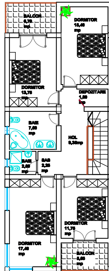
PLAN ETAJ Sc=110,00 mp Sd=215,10 mp
