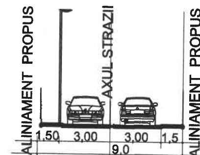
PROFIL STRADAL PROPUSE A-A
