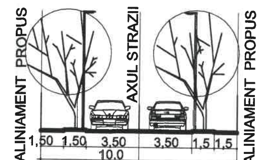
PROFIL B-B- STRADA PACII
