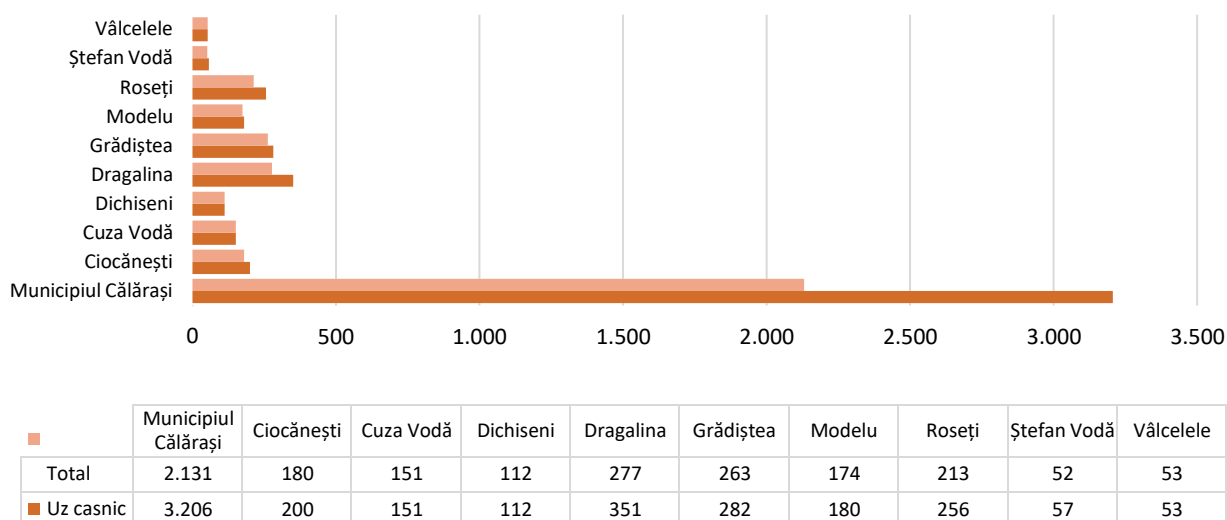
Figură 43: Cantitatea totală de apă potabilă distribuită consumatorilor în ZUF Călărași (mii m 3 ), 2019
